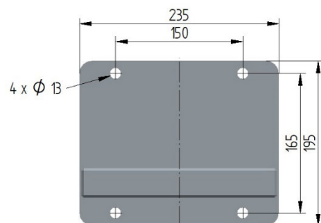
Wandkonsole DN 200mm
