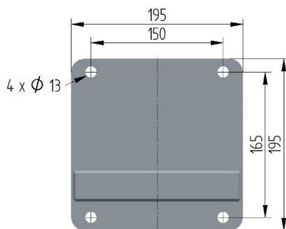
Wandkonsole DN 160mm
